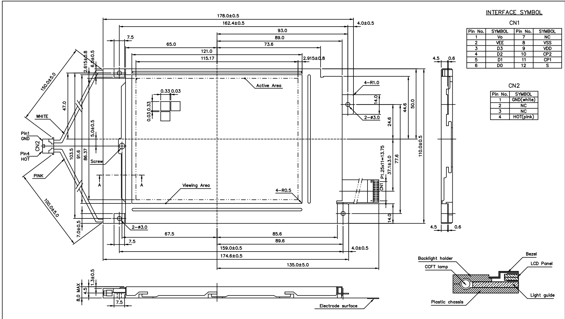
A-A' Section(Scale : 2/1)
