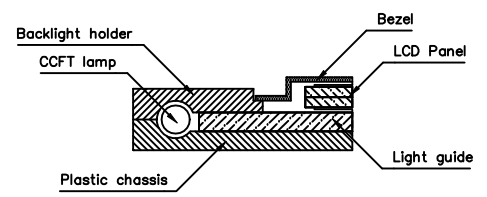
A-A' Section(Scale : 2/1)
