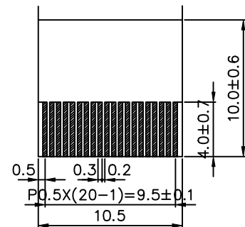
B DETAIL 1:3
